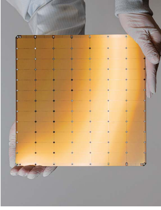
Abbildung 1: Chip des Cerebras CS-2-Systems: Rechenkraft und Speicher liegen nahe beieinander, das beschleunigt das Machine Learning. Foto: Cerebras Systems.
